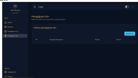
Gambar 9 Dashboard Karyawan
