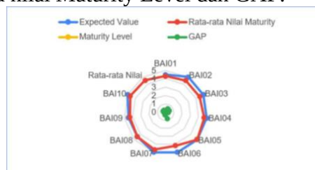
Gambar 2. Grafik Analisis Tingkat Maturitas dan Nilai GAP
