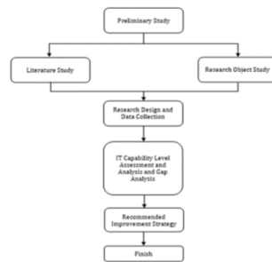
Gambar 1. Tahapan Penelitian
