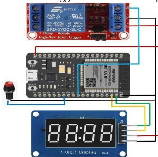
Gambar 2 Rancangan Rangkaian ESP32 dengan Relay dan Seven Segment
