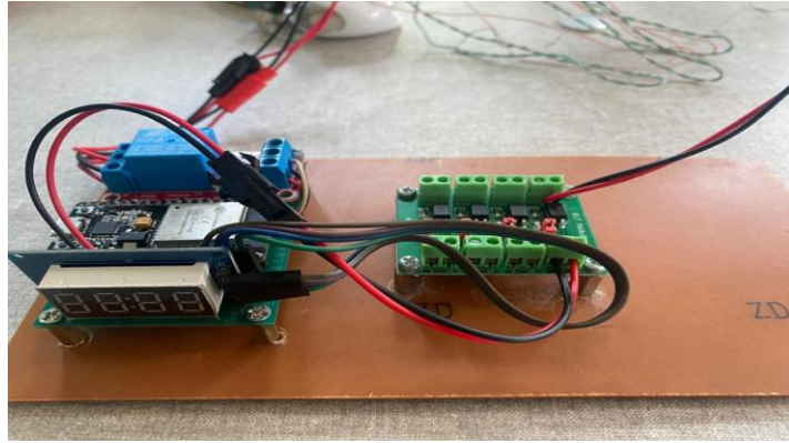
Gambar 6. Rancangan Changeover Otomatis Berbasis Waktu
